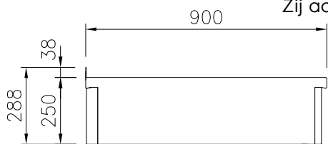
Zij aanzicht
